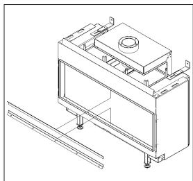
Rys. 15. Sposób demontażu szyby
