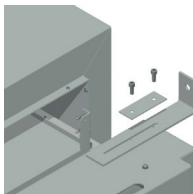
Rys. 3. Stopka poziomująca oraz regulowany uchwyt mocujący
