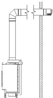
Rys. 5. Sposób wyprowadzenia koncentrycznego systemu kominowego
